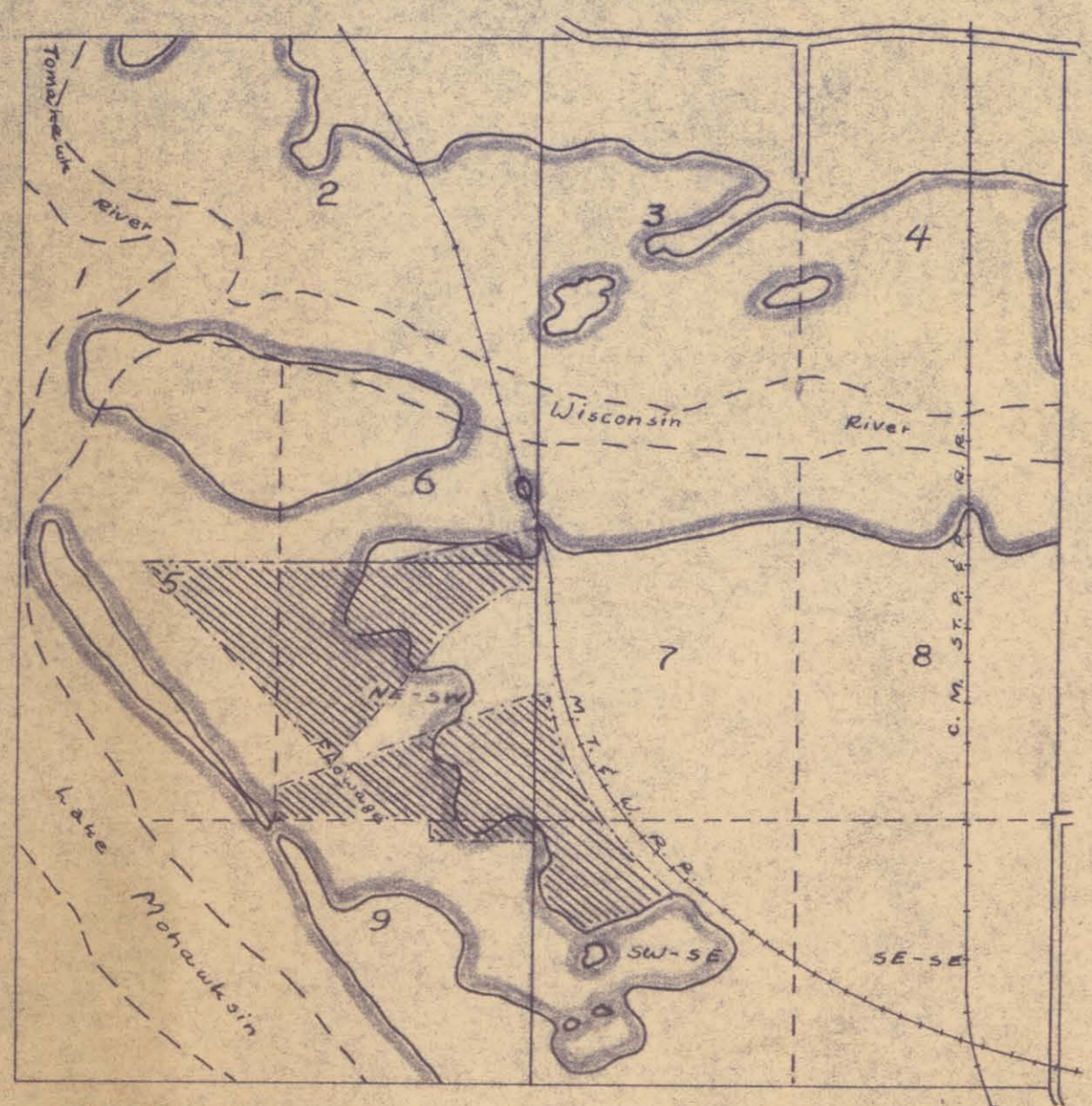
GENERAL LOCATION MAP SEC. 33, T. 35 N. R. 6 E.
