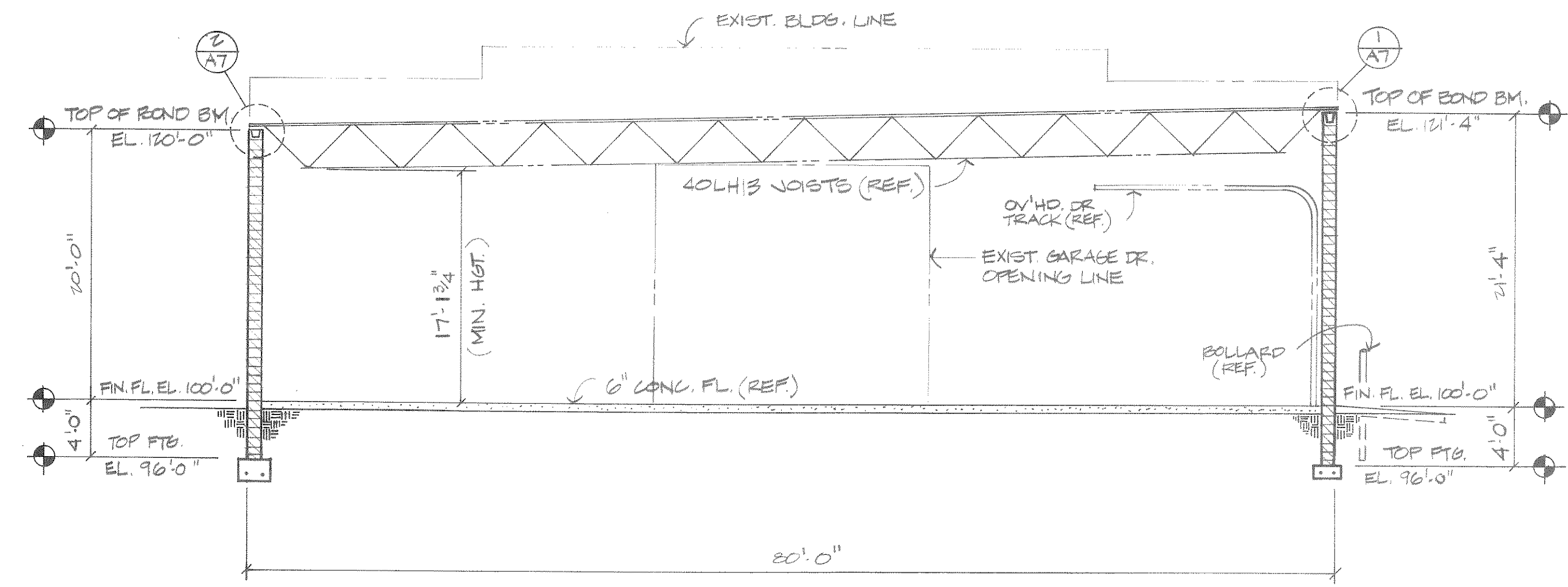
SECTION 2 A5 1/8"=1'-0"
