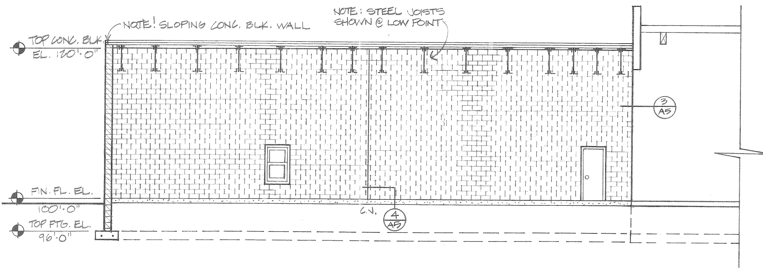
SECTION 3 A5 1/8"=1'-0"
