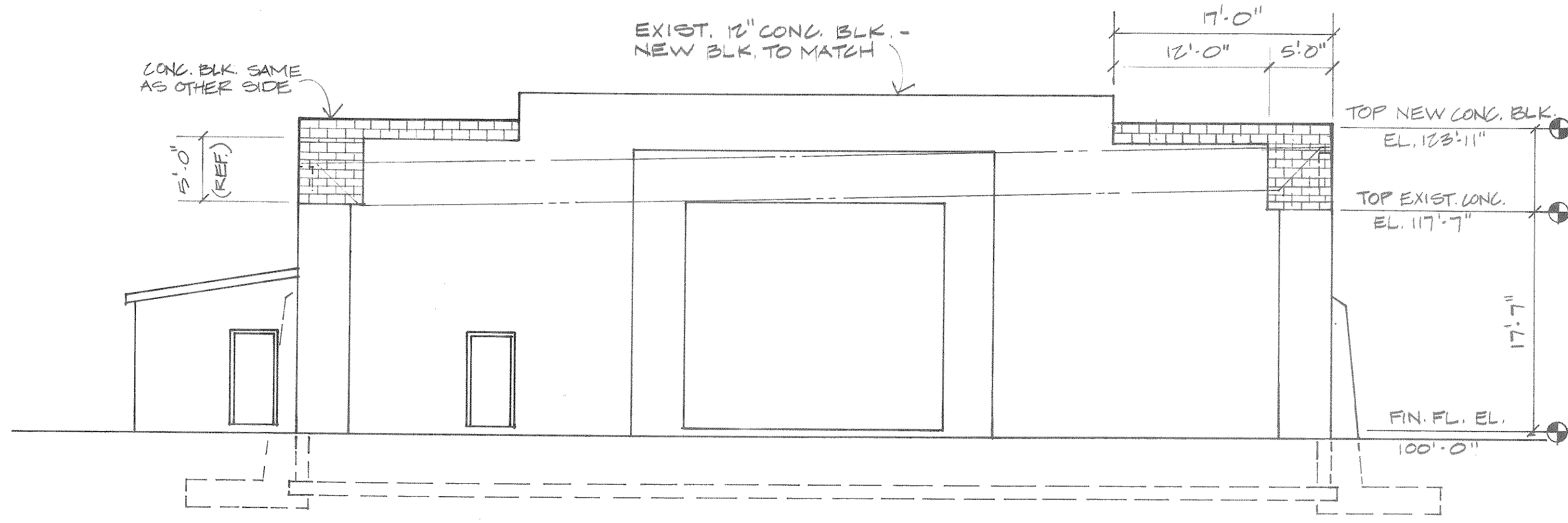
ELEVATION 1 A5 1/8"=1'-0"
