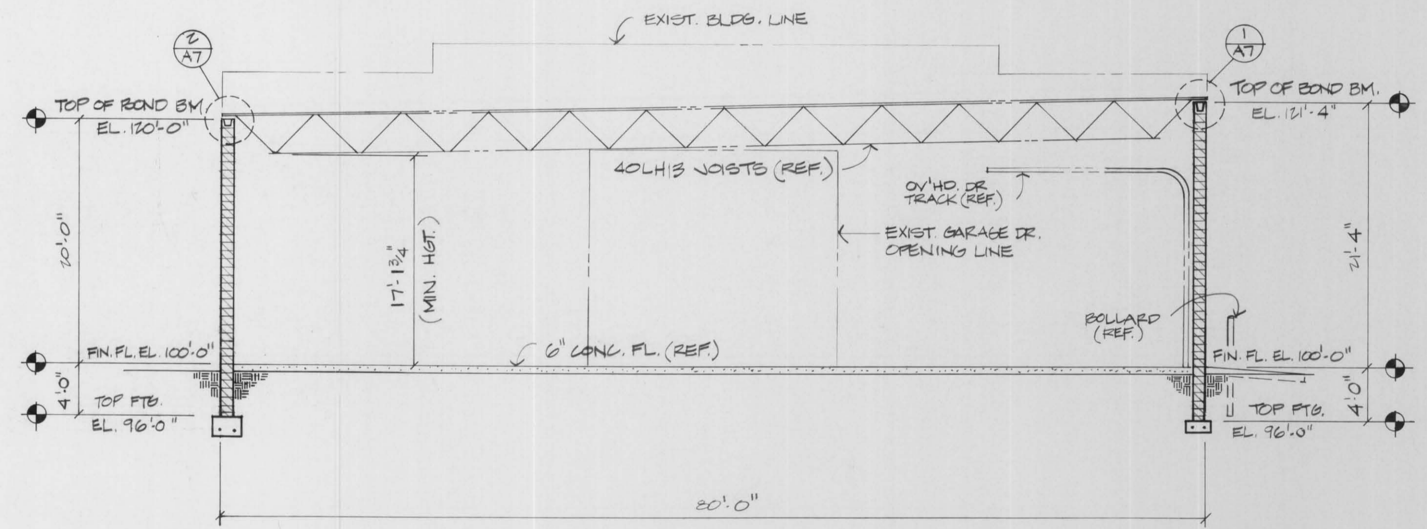
SECTION 2 A5 1/8"=1'-0"
