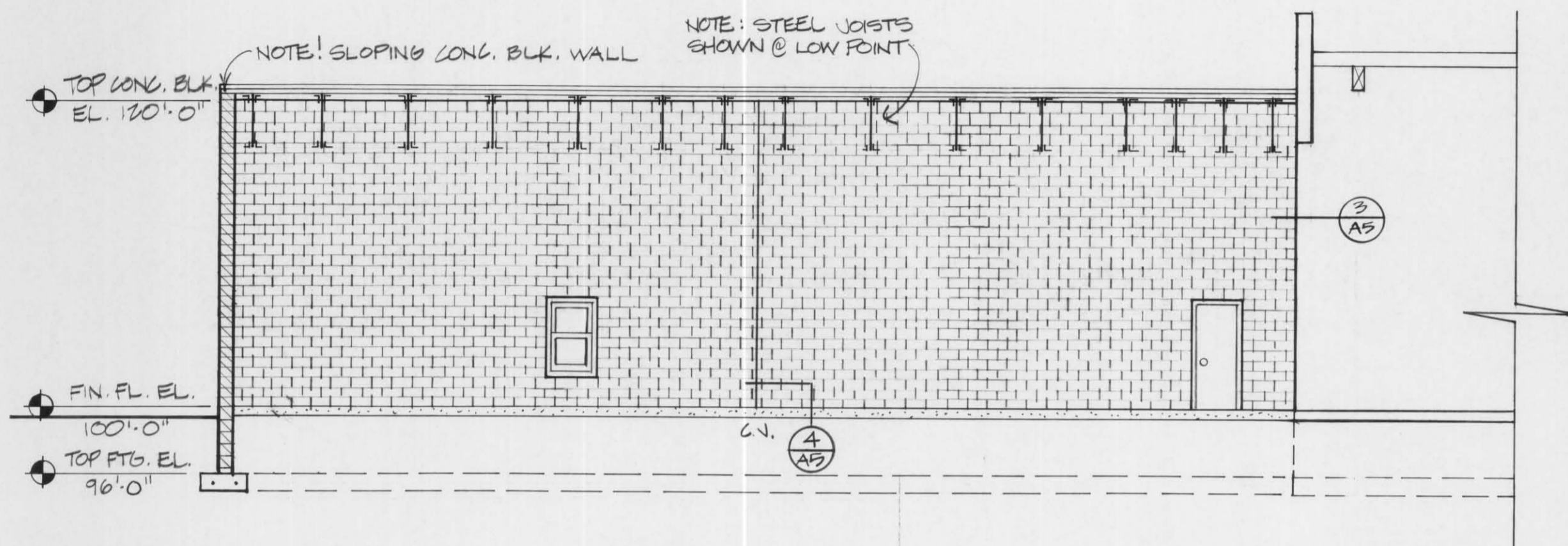
SECTION 3 A5 1/8"=1'-0"
