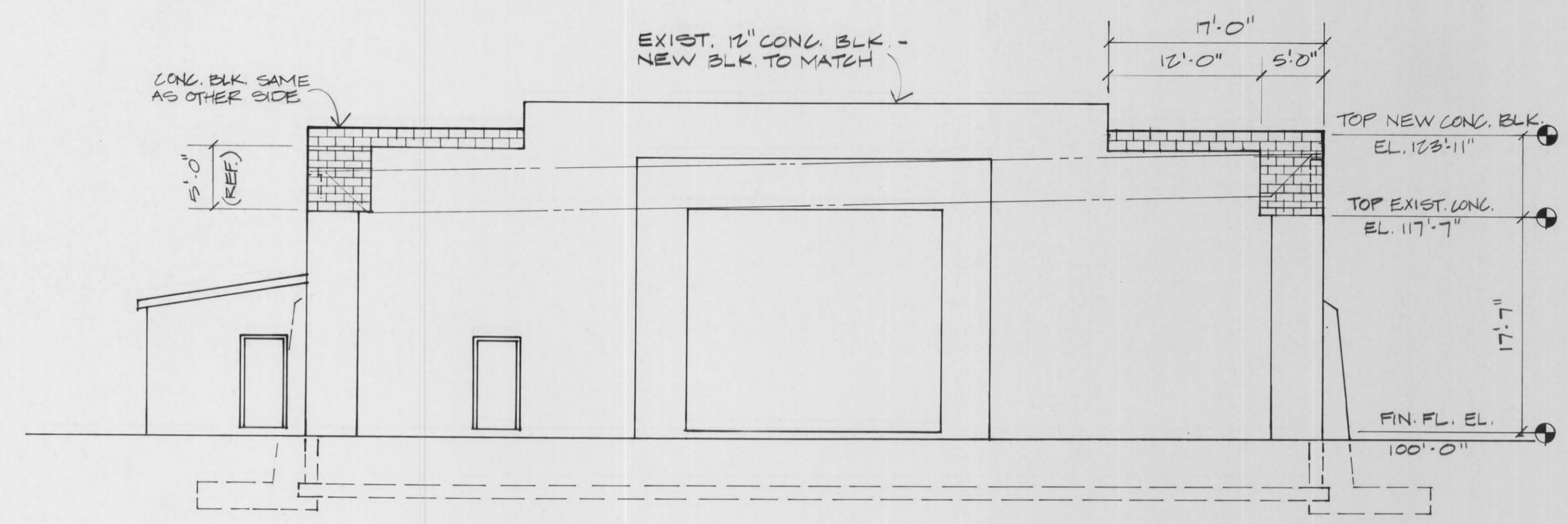
ELEVATION 1 A5 1/8"=1'-0"
